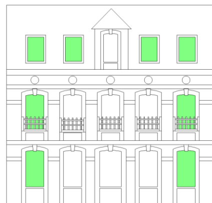
Exemple des nouveaux percements et fenêtres de toit respectant la symétrie et les trames du bâtiment ancien (en vert)
